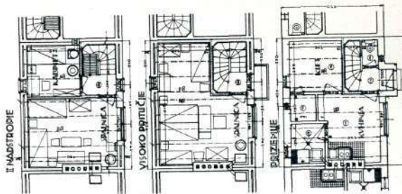
Iv. Vurnik: Načrt za delavsko enodružinsko hišo
