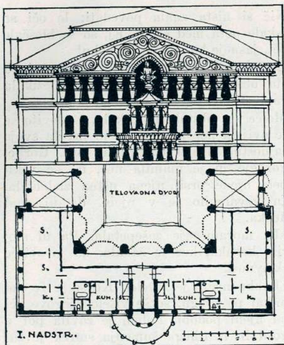
IVAN VURNIK: SKICA ZA FASADO II.
