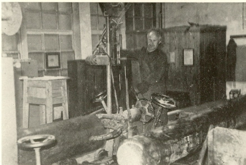
Razrez hlodovine na polnojarmeniku ESTERER
