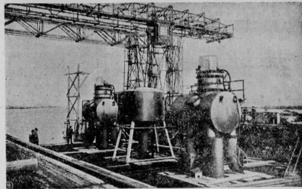
Slika 3. Vedno iznad vode gledajoči del kesona s tremi železnimi rovi, ki vodijo iz delovne dvorane, ki je globoko pod vodo. Na vrhu rorov vidimo prehodne kabine. Srednji rov in prehodna kabina sta za ljudi, oba stranska in dvojna pa za dvigavanje in odlaganje na dnu kesona nakopanega materiala. V ozadju vidimo veliki prevozni žerjav.
