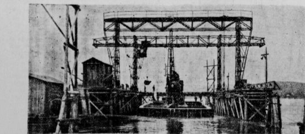
Slika 2. Ladja je potegnila iz zasilnega pristanišča v vodo spuščeni in plavajoči keson na sredo reke med oba montažna odra. Na sliki vidimo že, kako je keson potopljen med odroma, na katerih sta montirana dva vodoravna, prevozna in zelo močna žerjava. Na levi so na ladjah pripravljeni vsi potrebni stroji za mešanje betona, črpanje zraka itd.
