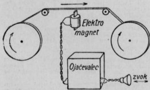
Skica aparata z zvočnim jeklenim trakom.
