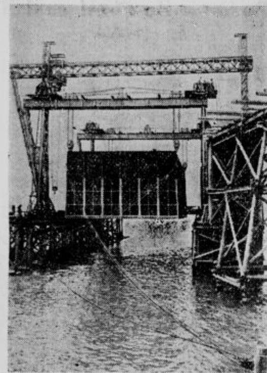
Slika 1. Zasilno pristanišče z odroma, na katero so raztovarjali ladje, ki so pripeljale sestavne dele kesonov. Med obema odroma so nato povprek zgradili oder, na katerem so sestavili keson. Slika nam kaže že sestavljeni keson, ki visi na močnem škripčevju. Prav na desni vidimo zasilni most, ki veže odra z bližnjim obrežjem.
