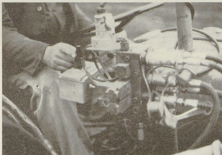
Ročica za štirismerno krmiljenje priključkov preko elektroventilov – podaljšana roka hmeljarja – omogoča hitro reagiranje
