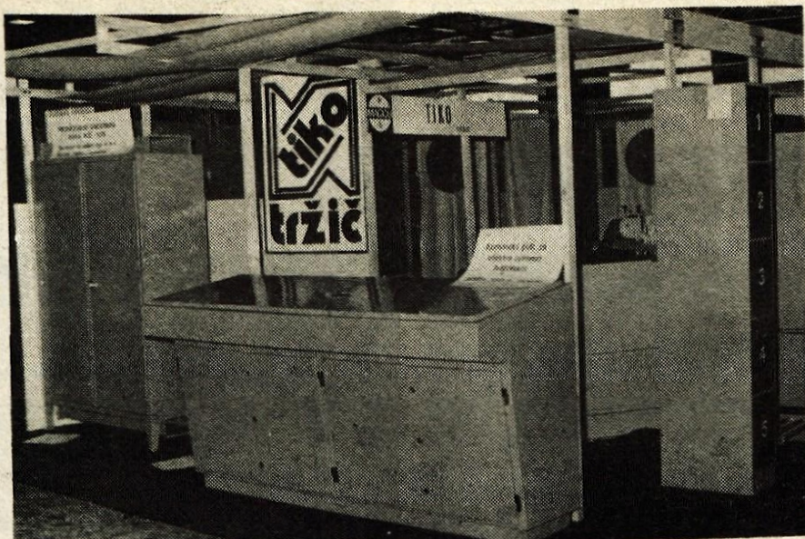
Tržiška industrija kovinske opreme Tiko v okviru poslovnega združenja Magos razstavlja kabelske omarice za električne priključke vseh vrst, omarice za orodje, galvansko kad z lovilem olja, komandne pulte, šoferske sedeže in prezračevalno garderobno omaro, ki je novost na našem trgu in prvi tovrstni izdelek v Jugoslaviji.
