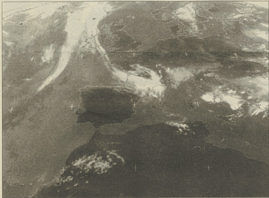
Formacija vremena nad zahodno Evropo
