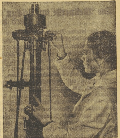
Einhängen der Objektpatrone in die geöffnete Schleusenammer des AEG-Übermikroskops.
