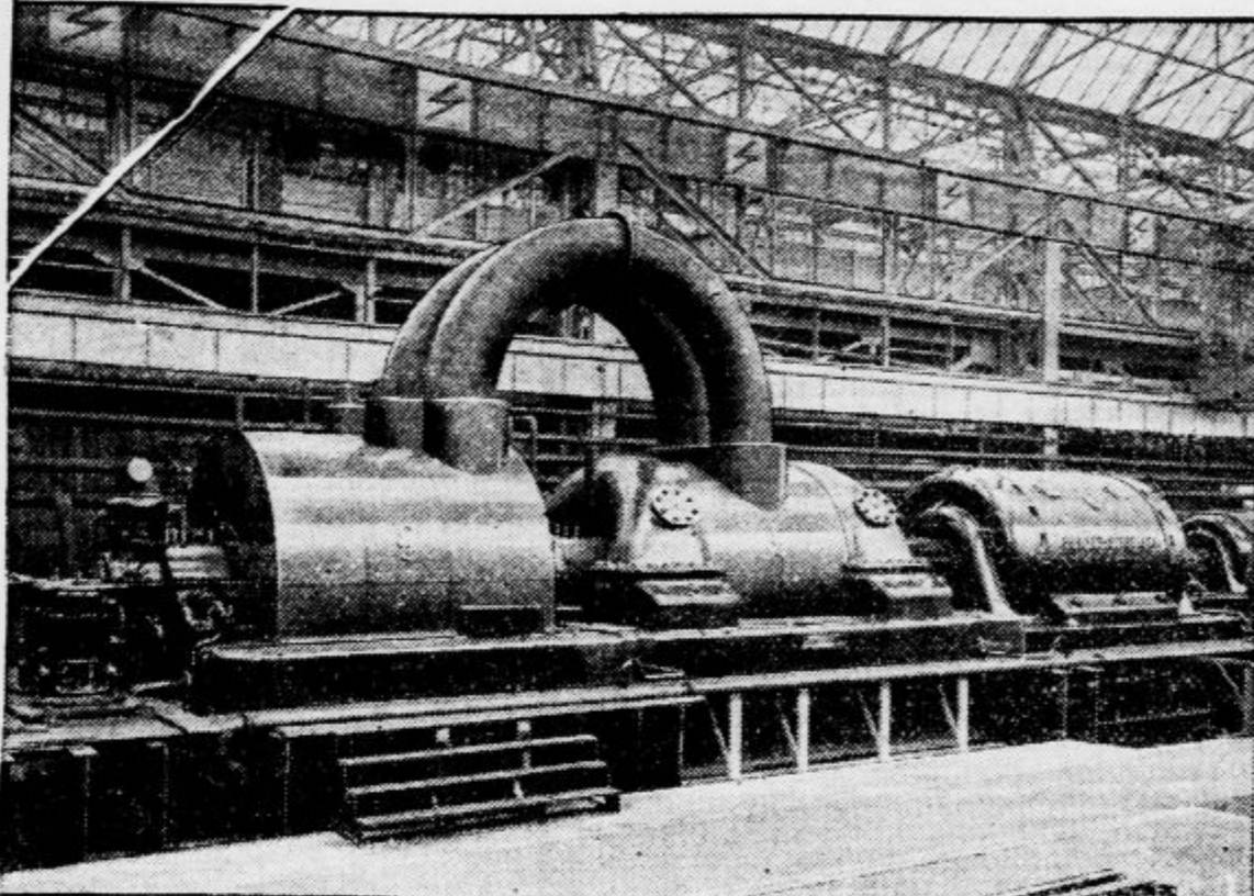
Rusija je naročila v Nemčiji ogromno kondenzacijsko turbino, ki napravi 3000 obratov v minuti in proizvaja kapaciteto 35.000 k. s. Naprava je direktno spojena z generatorjem za vrtilni tok. Rusija bo stroj namestila v eni svojih največjih elektrarn.
