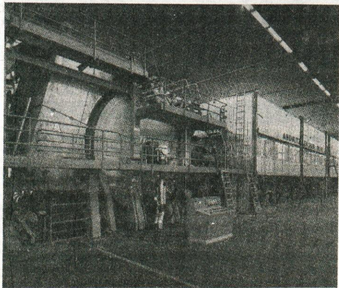
Papirnica Količevo, Kartonski stroj III.
