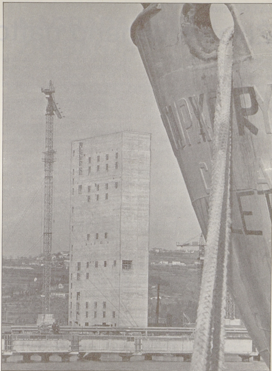
V koprski luki so lani začeli graditi silos za žitarice. To je ena največjih naložb v zadnjih letih v tem slovenskem pristanišču, zmogljivost silosa, ki bo končan do konca leta, pa bo 60.000 ton. Silos je tudi po gradbeni plati zahtevno delo, saj ga gradijo na mehki podlagi in so morali gradbinci zabiti kar 300 pilotov povprečno po 40 metrov globoko, da so pripravili dovolj trdne temelje (foto: Janez Zrnc).
