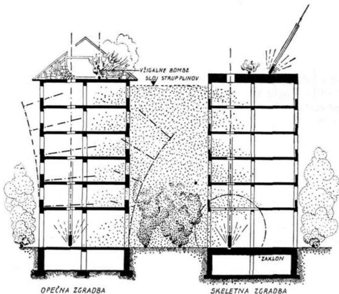
Prerez zgradb med zračnim napadom. Vpliv vžigalnih, razstrelilnih in plinskih bomb. Masivne zgradbe so manj odporne kakor skeletne zgradbe. (Po Gibrin et Heckly iz L'architecture d'aujourd'hui )
