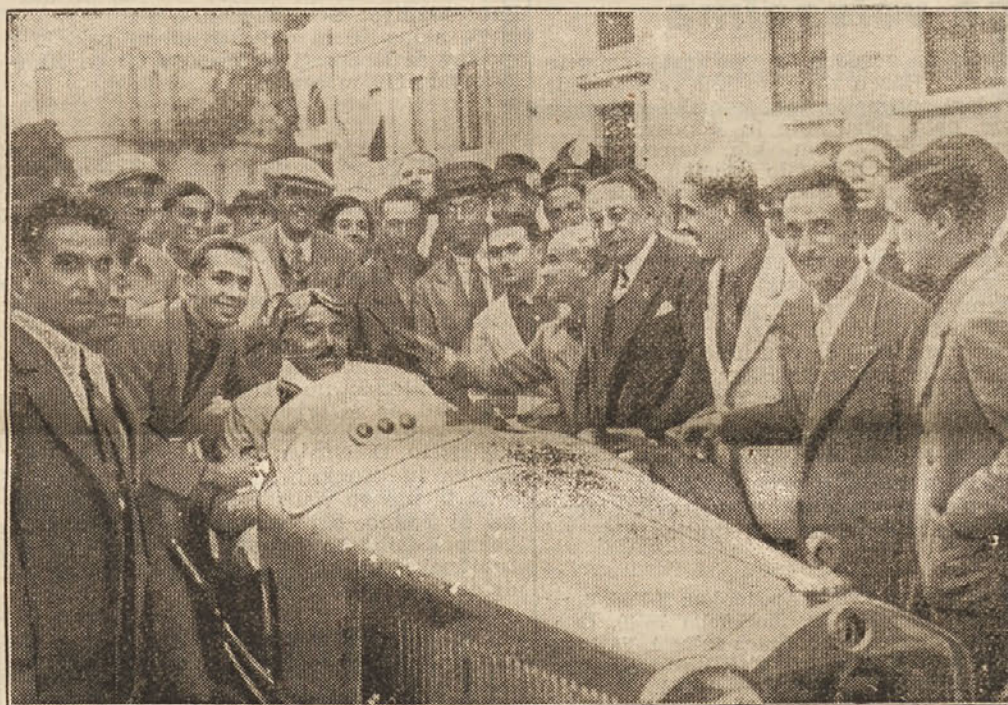
Italijanski profesor Ferraguti je pred kratkim prevozil 6000 km iz Rima čez Dunaj, Budimpešto, Krakovo, Varšavo, Berlin, Amsterdam, Bruselj, London, Pariz, Milan in zopet v Rim. Vozil se je s starejšo tipo Alfa-Romeo avtomobila, ki ga pa ne goni bencin, pač pa lesno oglje. Za vso vožnjo je porabil kuriva za okoli 600 dinarjev. Vozil je s povprečno brzino 95 km na uro. Ta poizkus dokazuje, da bo v avtomobilski industriji nastal popoln preokret, ki se ga bodo najbolj razveselili prijatelji avtomobilskega sporta in tudi naši oglarji. Slika kaže vozača pred odhodom iz Rima.
