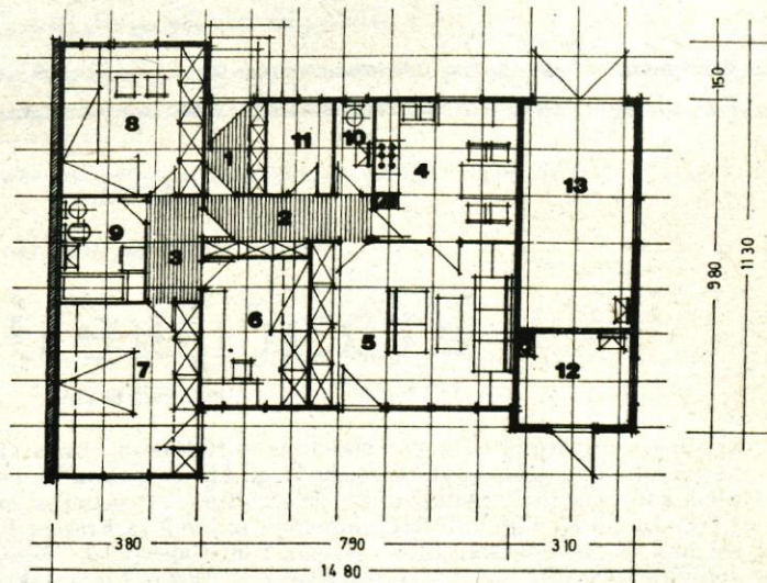
TLORIS PRITLIČJA B5 M 1:100
