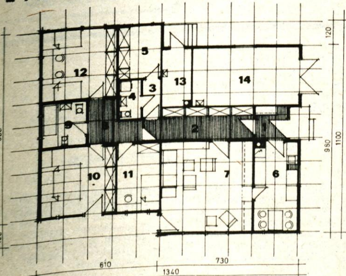
TLORIS PRITLIČJA B3 M 1:100
