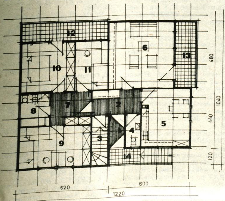
TLORIS PRITLIČJA B1 M 1:100
