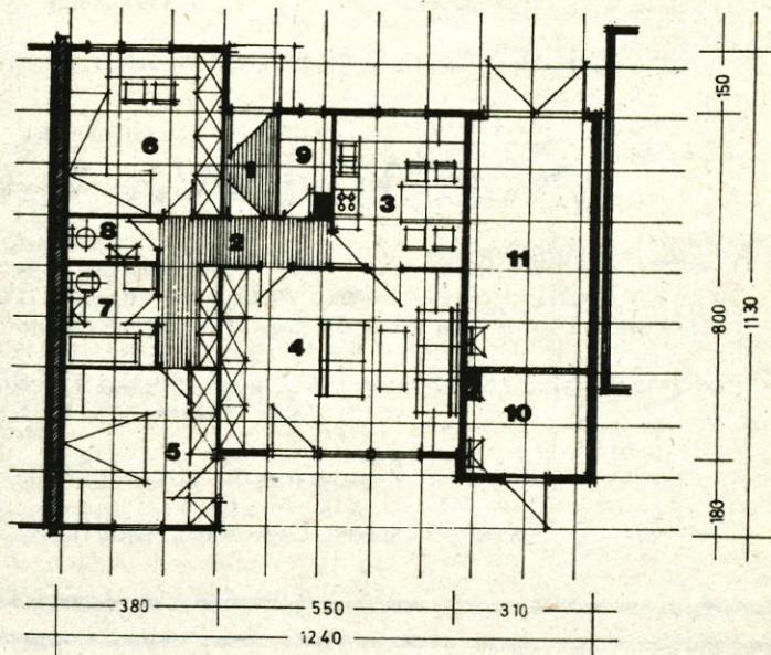
TLORIS PRITLIČJA B4 M 1:100
