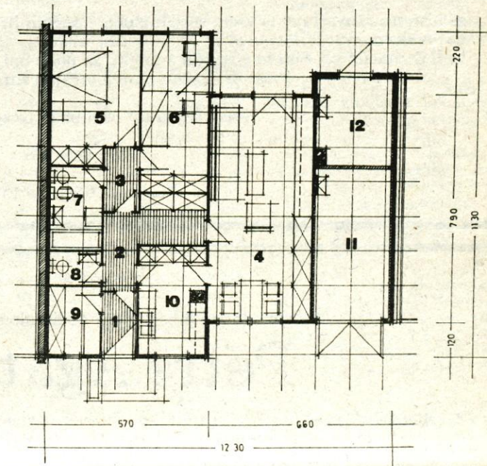
TLORIS PRITLIČJA B4a M 1:100
