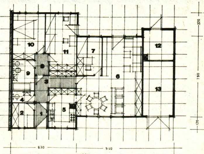
TLORIS PRITLIČJA B5a M 1:100
