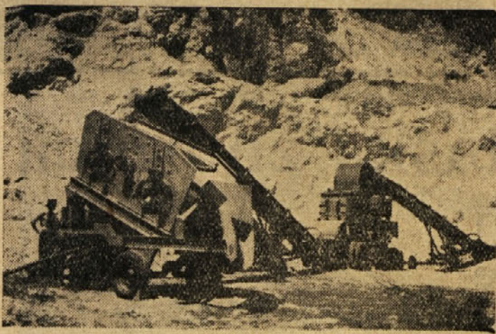
Droblilni in sejalni agregat, prevoznik, za drobljenje in sejanje, kompleten, je namenjen predvsem v gradbeništvu za pripravo sortiranega drobljenca. (Proizvod Strojne tovarne Trbovlje)
