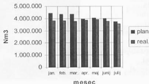
Poraba komprimiranega zraka v letu 2003
