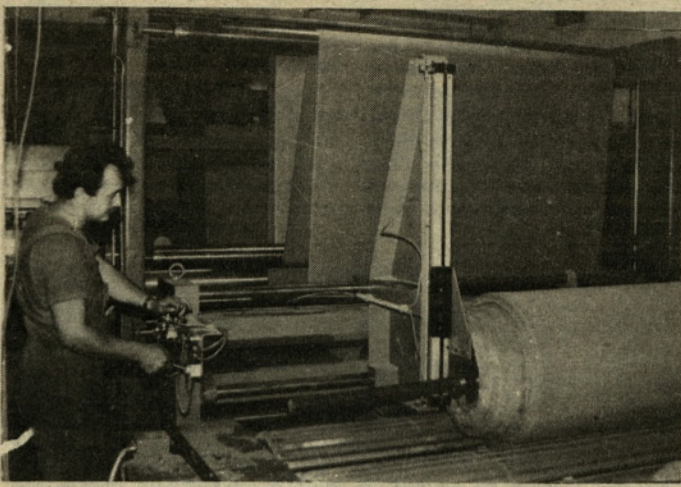
Stroj za proizvodnjo filca
