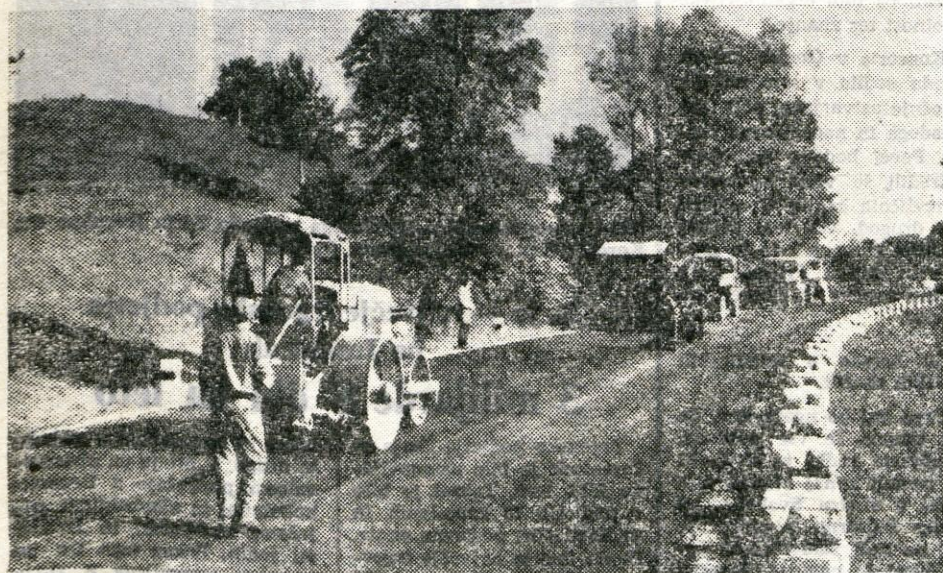
Delavci Cestnega podjetja iz Kranja zaključujejo dela na odcepu ceste Lesce—Bled. Te dni polagajo asfaltno prevleko in bo s tem rekonstrukcija tega odcepa zaključena, vožnja proti Bledu pa bo tako varnejša in prijetnejša. — Foto: F. Perdan
