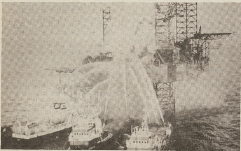
Gasilske protipožarne ladje z vodnimi topovi hladijo razgrete strukture mehiške vrtni ploščadi Abkatun 91 v zalivu Campeche, na kateri je pred tednom dni izbruhnil požar, a jim ga je uspelo omejiti brez človeških žrtev in z omejeno škodo (Telefoto AP)
