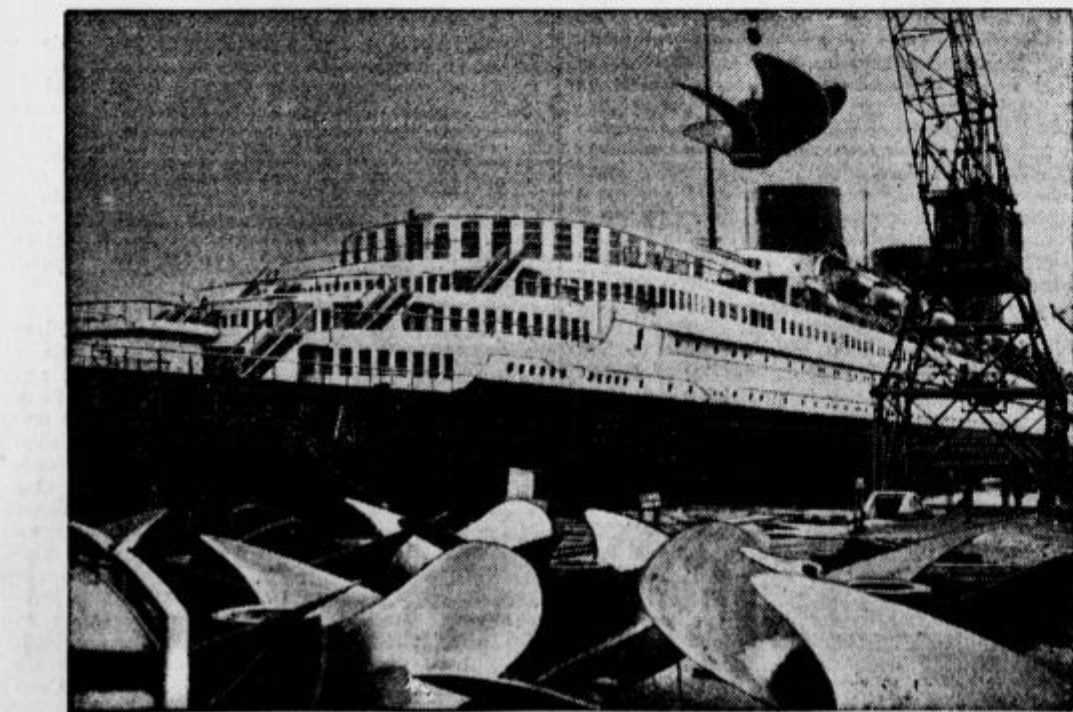
Za novo francosko ladjo »Normandie« ki v hitrosti tekmuje z angleško »Queen Mary«, so sedaj napravili mnogo lažje vijake, zaradi česar upajo, da bo ladja svojo hitrost lahko povečala. Te nove vijake, ki so težki samo 22 ton vsak, namestu 26 ton, kakor doslej, montirajo na ladjo.
