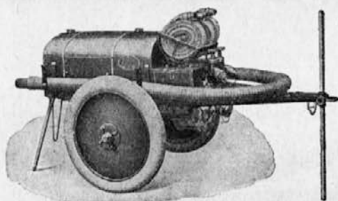
Lahka, dvokolna motorna brizgalnica z 16/18 HP motorjem, dobava vode 800 l v minuti, pritisk do 12 atm.
