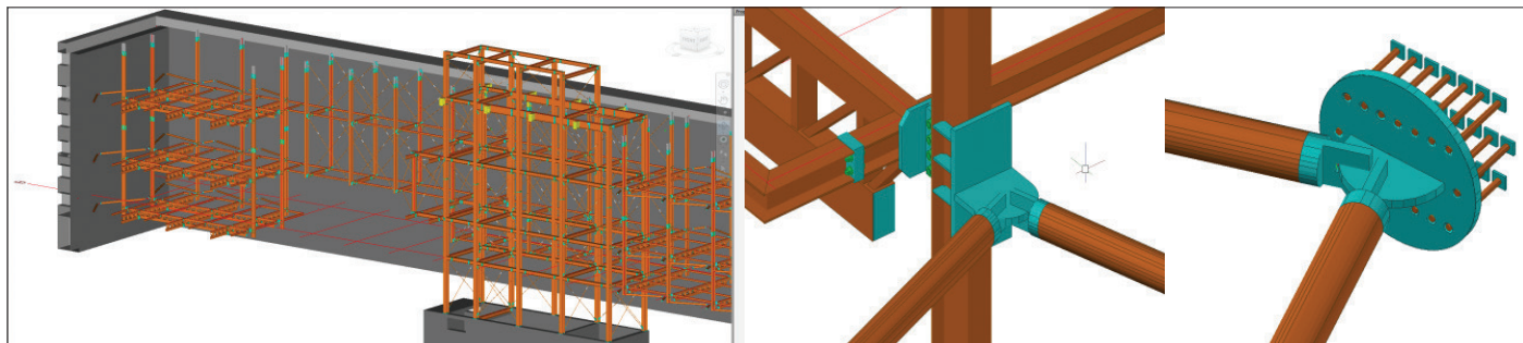
Slika 9 • Jeklena konstrukcija medetaž in detajl priklapa diagonalnih razpor.
