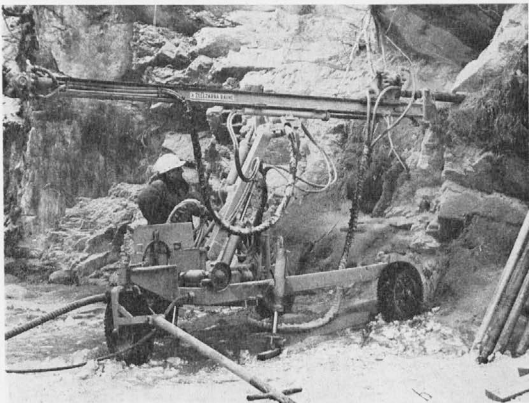
Vrtalna garnitura RGVS
