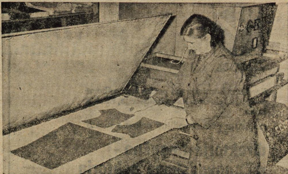
Fiksiranje medvlog na tkanine na fiksirni stiskalnici pri temperaturi 160 stopinj Celzija in pritisku 450 kilopondov
