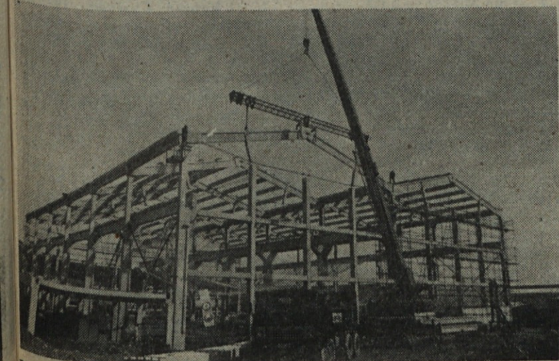
Montažna hala GH-6
