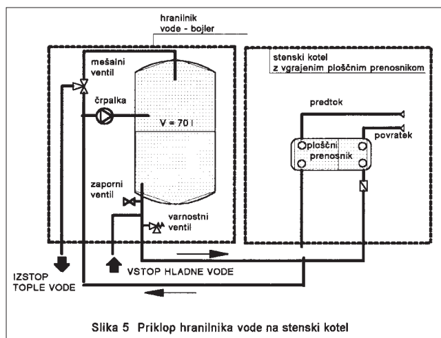
Slika 5 Priklop hranilnika vode na stenski kotel
