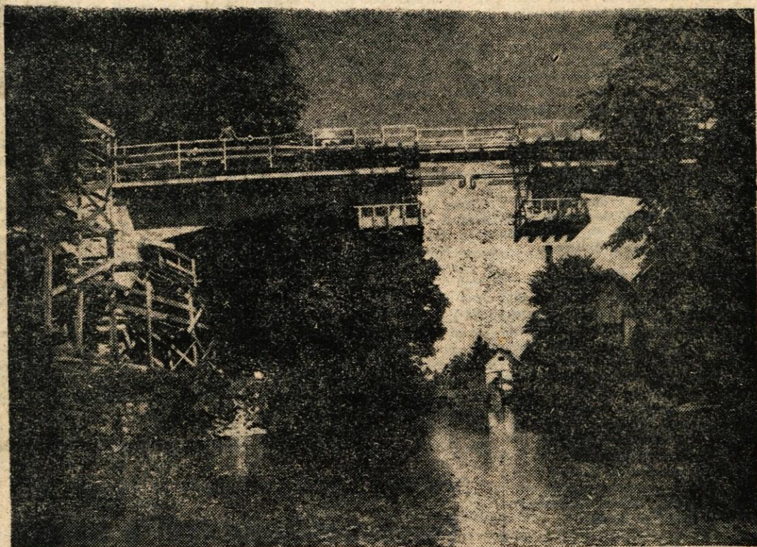
SGP Tehnik iz Skotje Loke se je prvo v Jugoslaviji lotilo nove gradnje mostu. Most čez Somo v Skotji Loki gradijo pa delih - brž ko je določena dolžina betonskega mostu dovoli, dogradijo spet nov del mostu (na sliki)
