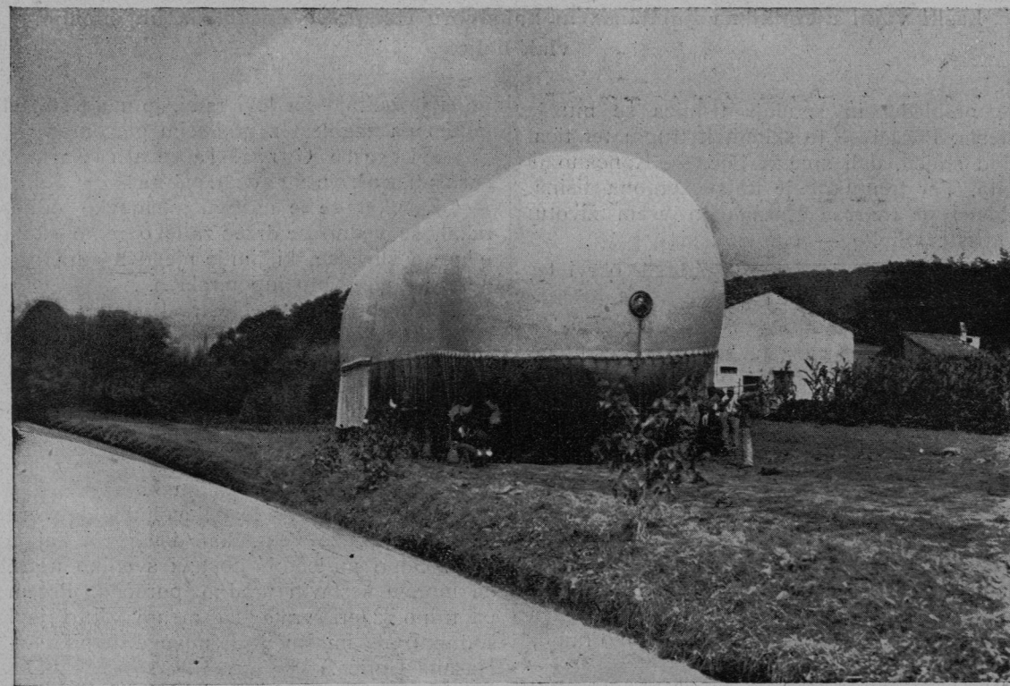
Z goriške fronte: Naš opazovalni zrakovplov, skrit za goriško vasico, predno se dvigne opazovat laške naklepe.
