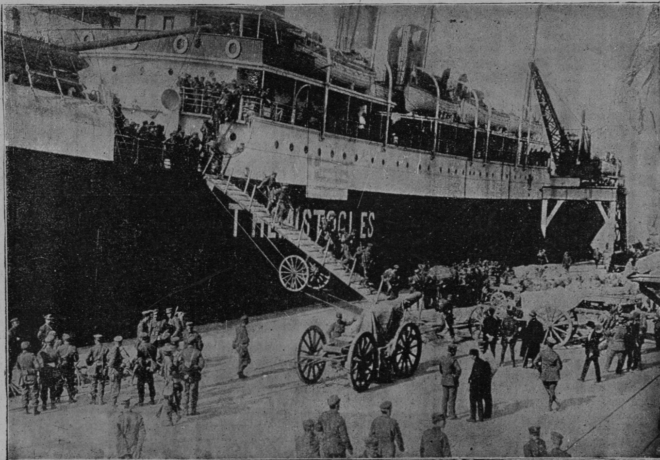
Izkrcavanje čet pri Solunu.
