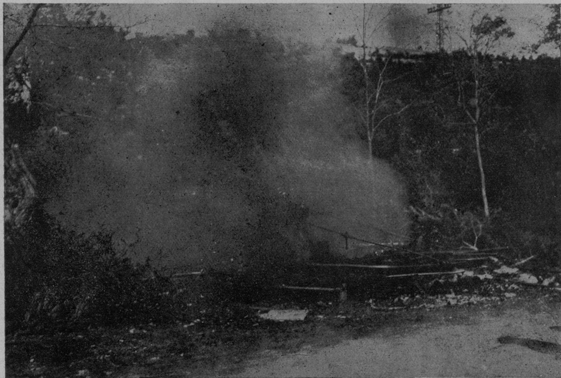
Z goriške fronte: Ogronomni dim po strelu iz našega 30.5 cm topa. Te najboljše topove na svetu je dal napraviti in uliti naš šef generalnega štaba pl. Hötzendorf.
