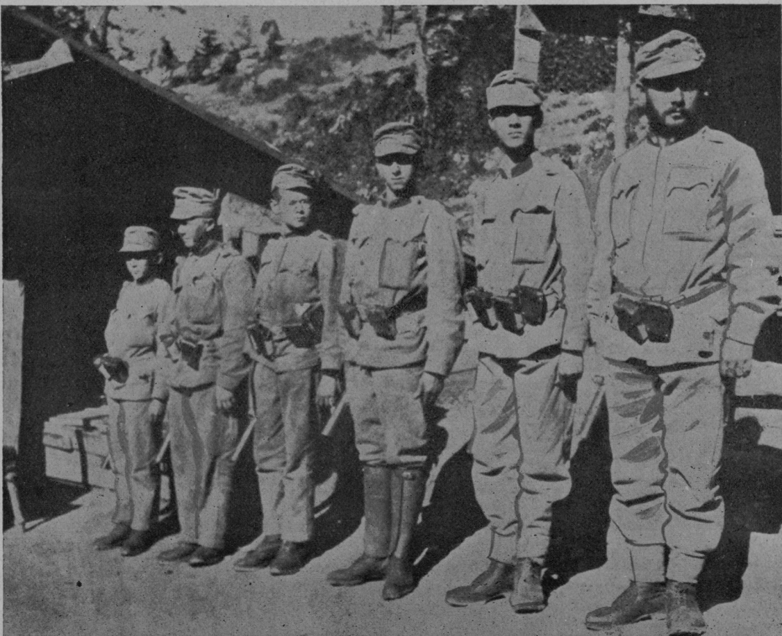
Za hrabrost odlikovani slovenski mladostrelci.
