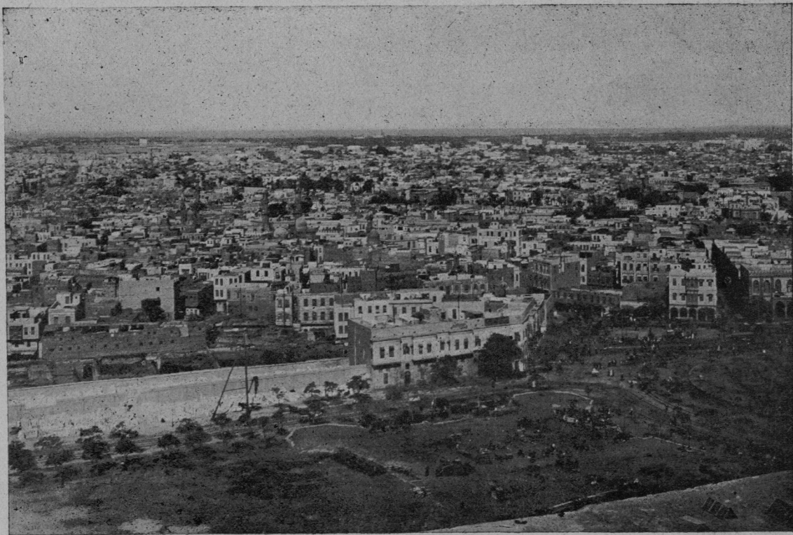
Glavno mesto Egipta, Kajira, ki ga hočejo Turki osvoboditi iz angleške oblasti.
