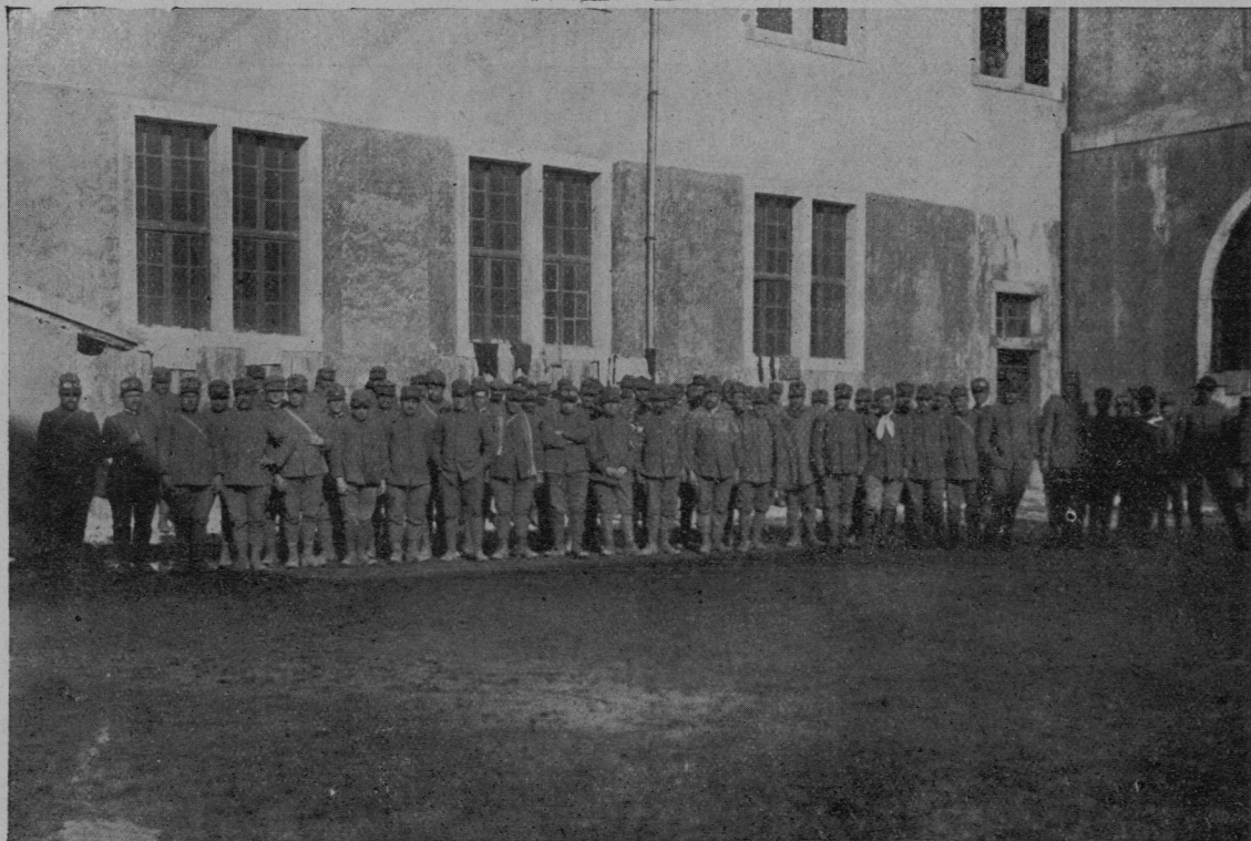
Laški vojni ujetniki na dvorišču ljubljanskega gradu pri jutranjem raportu.
