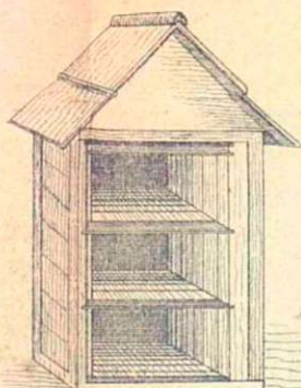
Fenster. Okence. Halbständer mit abnehmbarem Dache Nr. 3. Vispki panj s premakljivo streho št. 3.
