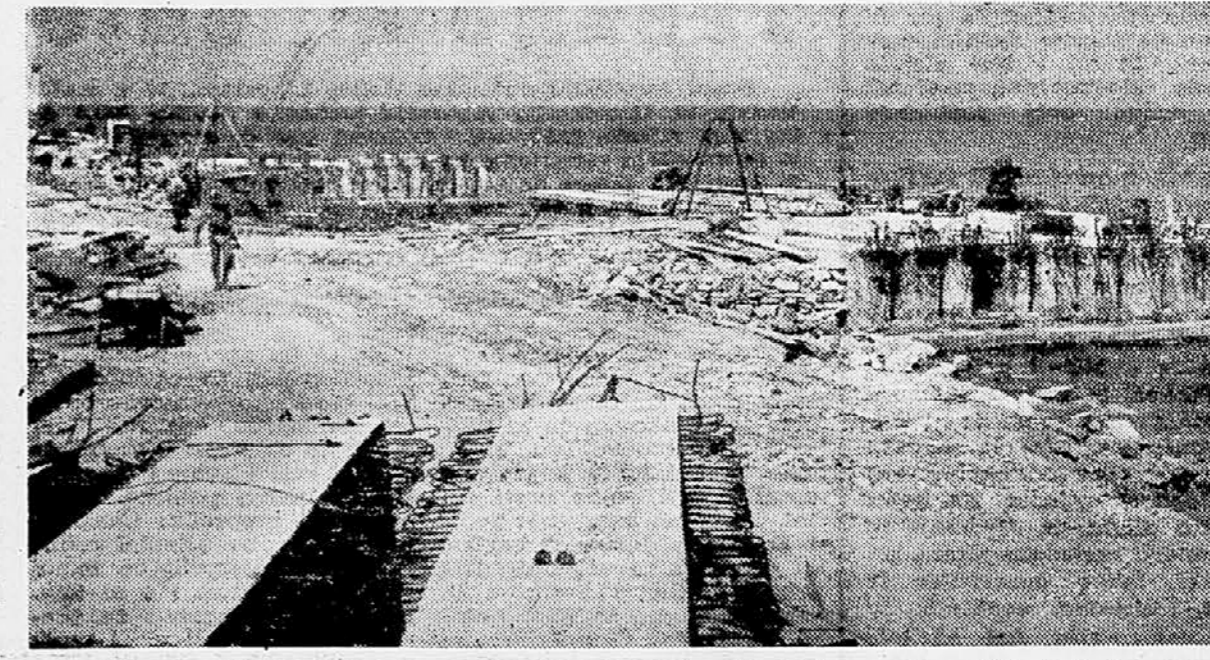
Pogled na gradilišče luke 12. avgusta: »Zmeda« betonskih blokov, nosilcev, železja in kamenja.
