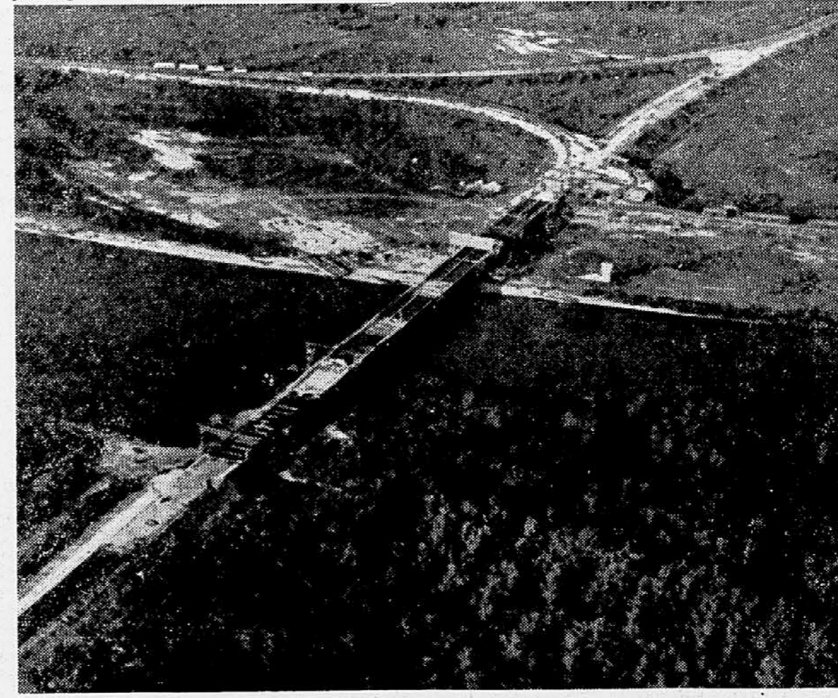
Največji objekt na avtomobilski cesti — most čez Savo pri Samoboru. Dolg je 320 m. Konstrukcija je izdelala mariborska »Metalna«. Po mnenju strokovnjakov je bila postavitvev mostu rekordna, ker so ga šele aprila letos začeli delati v tovarni. V sredo so pričeli most betonirati. (Foto: Stanko Vrnčič)
