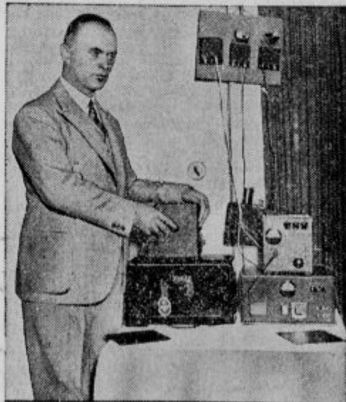
Brezčično naznanjanje požara. Nemški policijski stotnik Ristow je izumil napravo, s katero je mogoče brezčično naznaniti požar.
