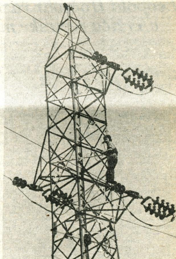
Obnova 35 kV daljnovoda Jesenice — Kranjska gora, ki je bil kamen spotike zlasti zadnjo zimo.
