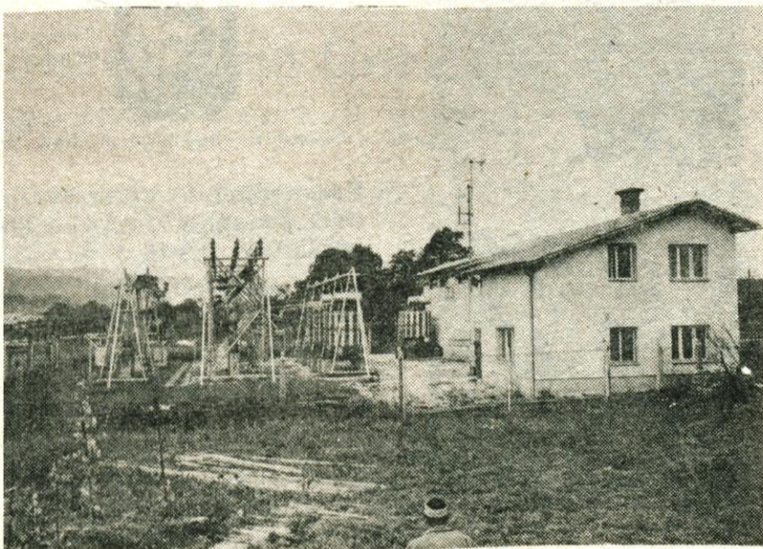
Razdelilna transformatorska postaja v Radovljici ob kateri bo v kratkem zgrajena nova 110 kV RTP. Gradnja se je že začela.
