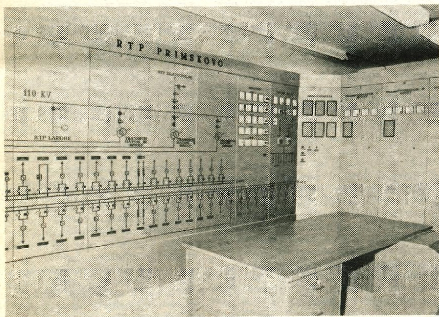
Komandna plošča 10 in 20 kV stikališča nove razdelilne postaje na Primskovem
