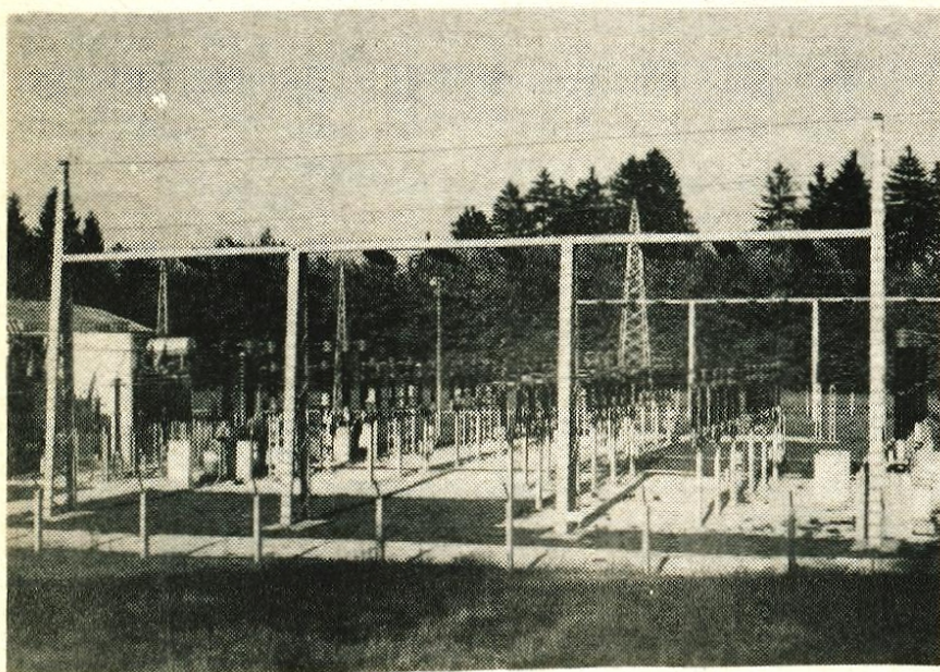
110 kV razdelilno trafo postaja na Laborah, ki napaja predvsem kranjski industrijski bazen.
