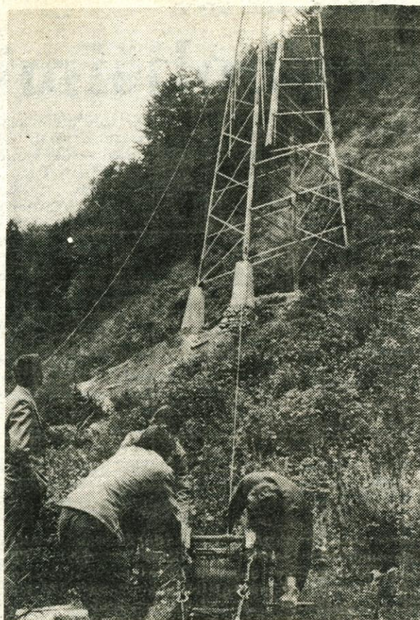
Gradnja 110 kV daljnovoda Bled — Bohinj, ki bo izredno pomemben za boljšo preskrbo z električno energijo v bohinjskem kotu. V začetku bo obratoval z močjo 35 kV in bo nadomeščal dotrajani daljnovod, ki poteka prek Pokljuke in Jelovice v Bohinj.
