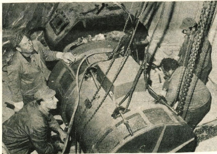
Montaža generatorja v hidroelektrarni Soteska pri Bohinju TOZD Elektro Sava Kranj. Elektrarna bo zgrajena na temeljih nekdanje žage in bo vključena v sredjenapetostno omrežje bohinjsko-blejskega območja. Moč nove elektrarne bo 400 kVA.
