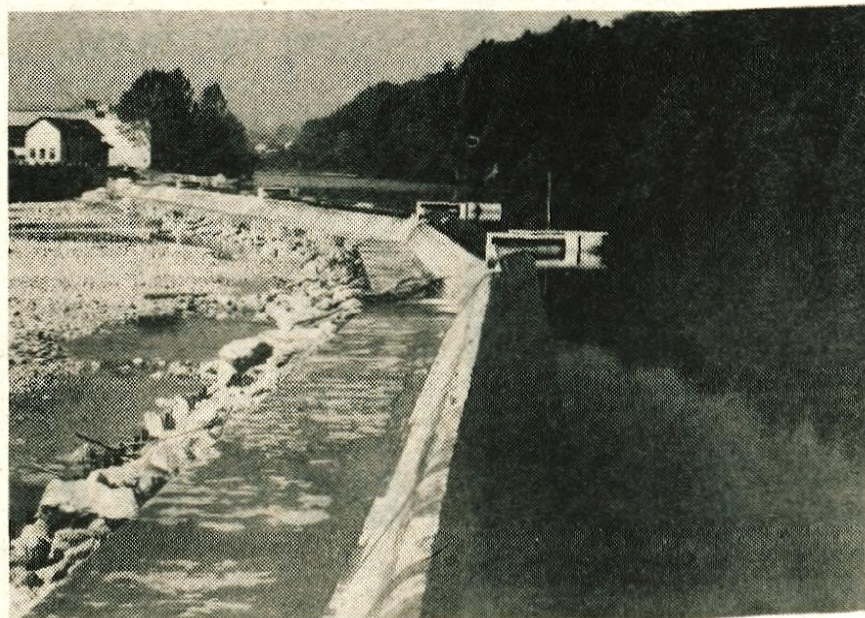
Novost na področju jezovne gradnje za hidroelektrarne je plavajoči nastavek za uravnavanje vodnega režima. Takšen nastavek ima elektrarna Sava v Kranju.
