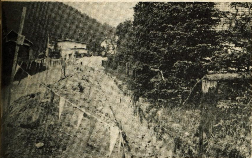
Vodovod v Ratečah za nove žičnice — Delovna organizacija Kovinar Jesenice letošnje poletje opravlja obsežna gradbena dela za postavitev novih žičnic in vlečnic v Kranjski gori. Tako so morali skopati rove in položiti vodovodne cevi tudi v Ratečah. — Foto: D. Sedej
