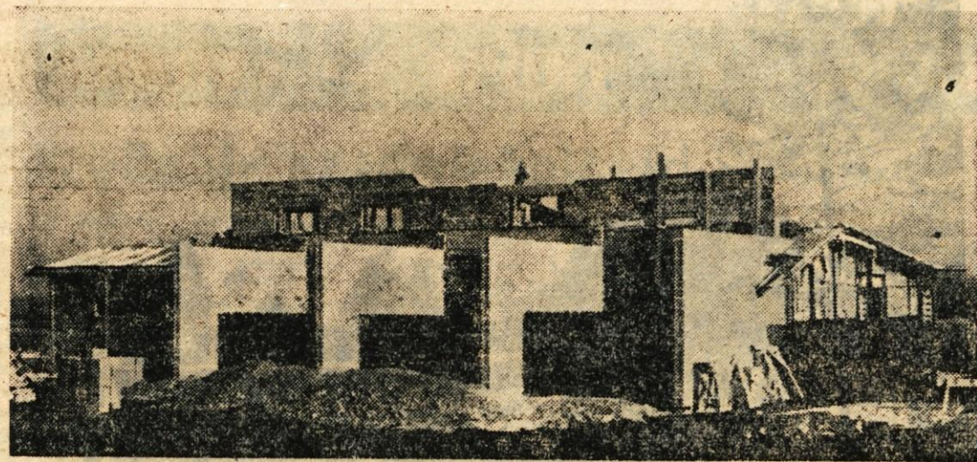
Na Zlatem polju v Kranju gradijo razdelilno transformatorsko postajo, ki jo bosta napajali z električnim tokom hidrocentrali v Mostah pri Zirovnici in v Medvodah. Gradnja v prvi fazi bo veljala okrog 90 milijonov dinarjev. Del zneska bo prispeval Elektro Kranj iz lastnih skladov, ostalo pa bodo krili s krediti in s prispevki kranjskih podjetij. Trafo postaja bo imela dva transformatorska motorja s skupnim učinkom 12 MVA, in bo namenjena razdeljevanju električne energije potrošnikom v Kranju — S. S.
