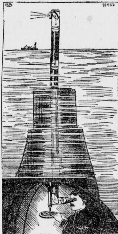
PERISKOP AMERISKEGA PODMORSKEGA ČOLNA.
