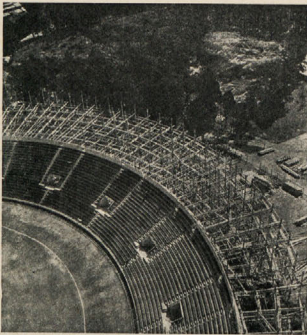
Olimpijski stadion v Helsinkiju med delom.
