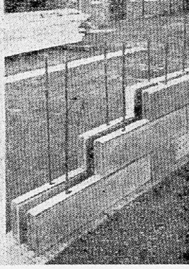
Neka angleška gradbena tvrdka je patentirala nov izum. Gre za posebno vrsto opeke, ki se nataka na jeklene palice, tako da ni treba zidati več z malto. Taka gradnja je veliko hitrejša, razen tega pa je mogoče zgradbo s takim zidom porušiti in prestaviti brez težav. Enodružinska hiša se more postaviti s to opeko v 24 urah.
