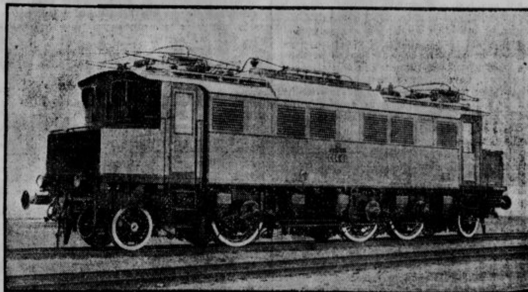
Najhitrejša električna lokomotiva v Evropi, ki so jo pravkar preizkusili na nemških državnih železnicah. Vleče sedem velikih potniških voz z brzino 151,5 km na uro.
