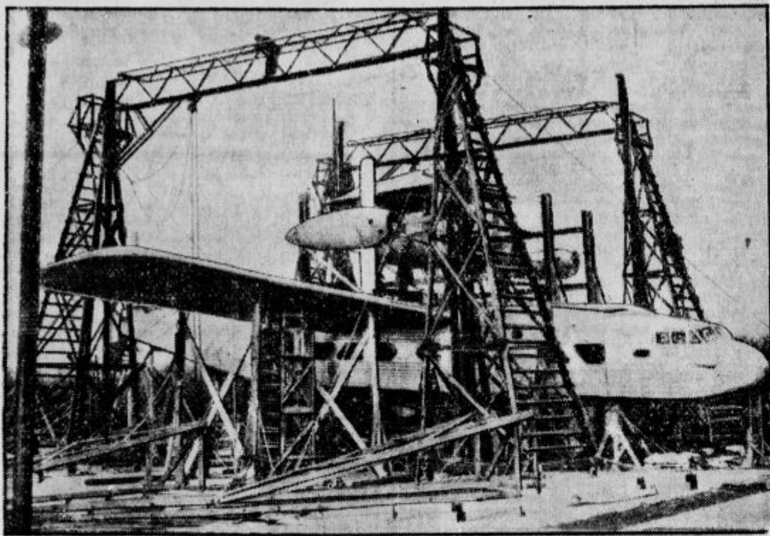
V tovarni letal v Rochesterju na Angleškem gradijo štirimotorno letalo, ki ga bodo uporabljali za potniški promet. Na njem bo prostora za 43 oseb. Čeprav ni to pomorsko letalo, se trup gradi, kakor da bi šlo za hidroplan
