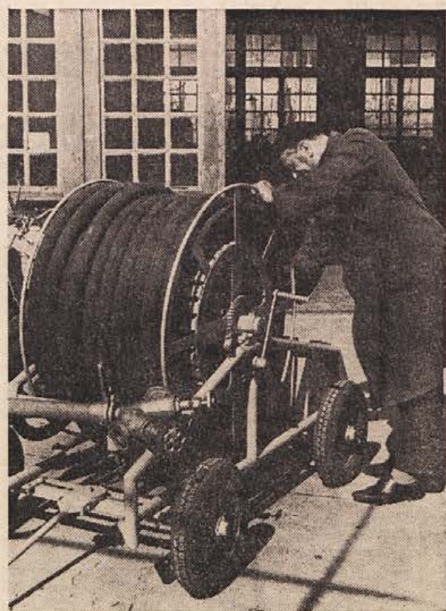
Črnomaljski mehanik Franjo Oblak je v svoji delavnici izdelal za potrebe krajevne skupnosti stroj za pranje mestnih ulic. V kratkem bo stroj dokončan. Pravi, da bodo z njim prvi škropili pred prvo-majskimi prazniki. — (Foto: R. Bačer)
