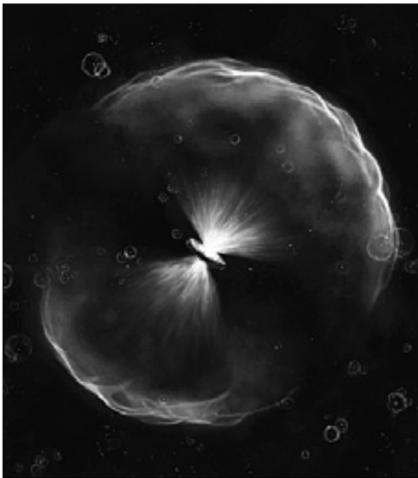
Kvazar s črno luknjo z maso dveh milijard naših Sonc
