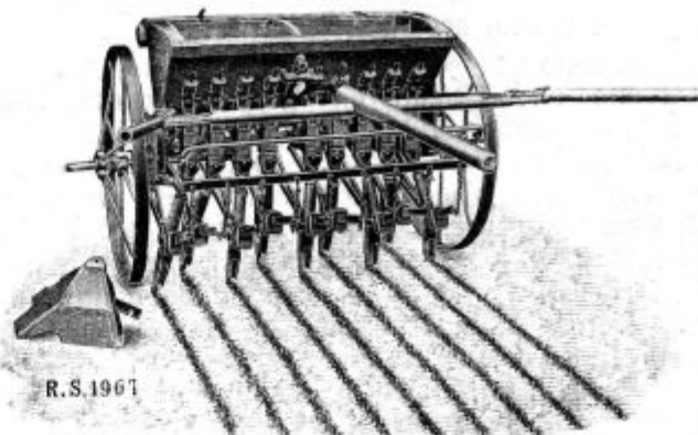
Slika 42. Ročni sejalni stroj. Teža 120 kg. Dnevno poseje 2 do 2.50 ha.
