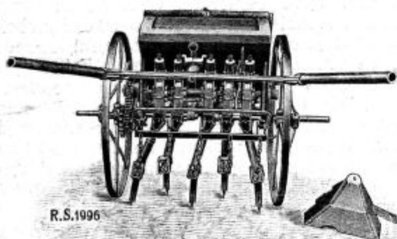
Slika 41. Ročni sejalni stroj. Teža 81 kg. Z njim posejemo 1.25 do 1.75 ha na dan.
