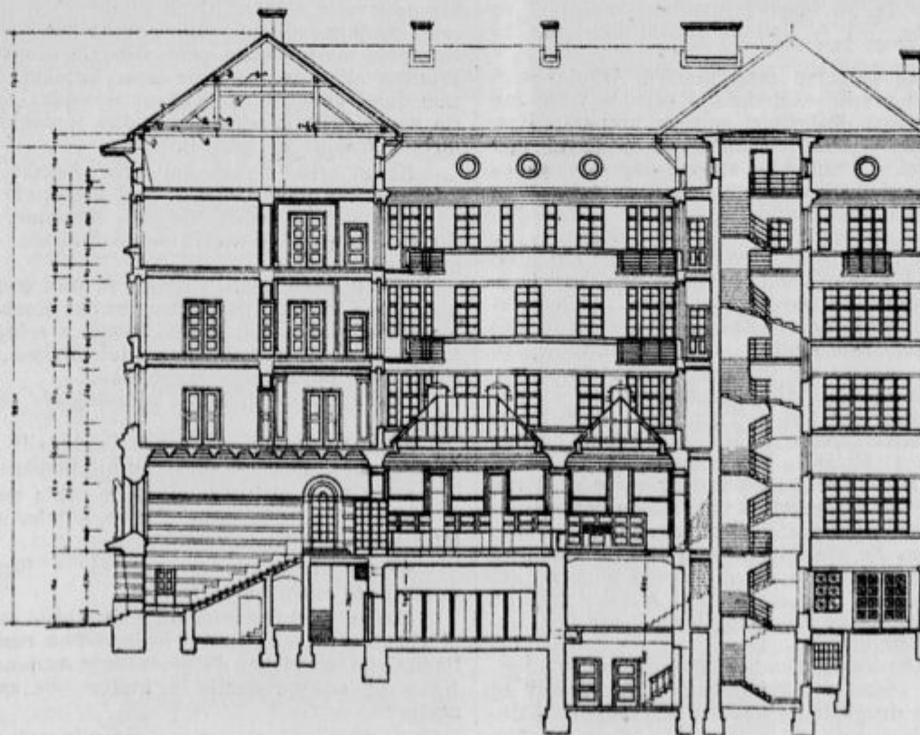
Načrt palače poštne hranilnice v Ljubljani v prerezu.
