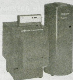
Vitola-comferral 15 do 63 kW nizkotemperaturni ogrevalni kotel na olje/plin, tudi kot paket z ogrevalnikom sanitarne vode
