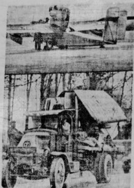
Ameriška vojna mornarica si je zgradila nov tip letala, ki ga bodo lahko spravili tudi na podmorske čolne. Letalo se da zložiti in v treh minutah zopet pripraviti za polet. Leti z brzino 160 km. Spodaj letalo na vojaškem avtomobilu
