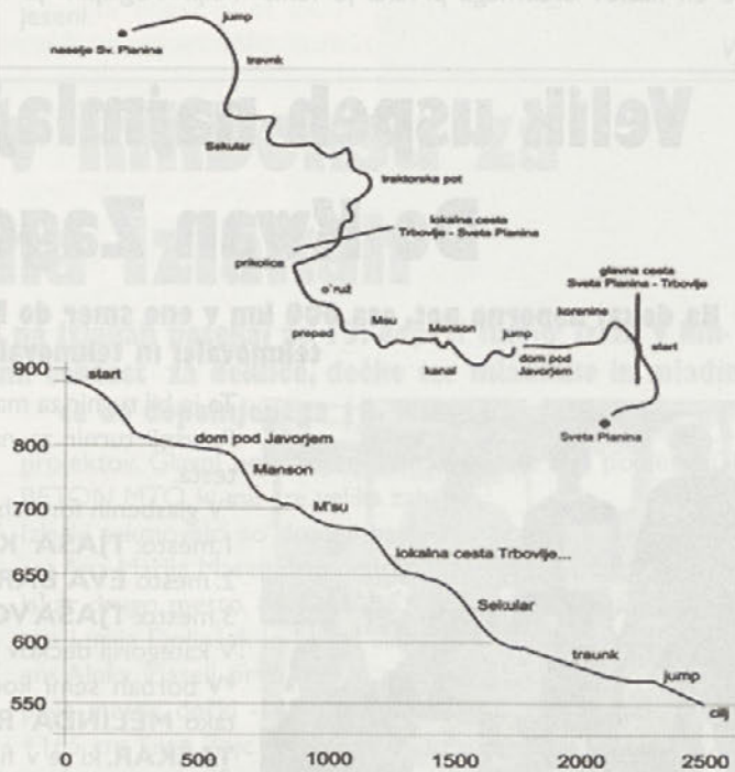
Shema proge za downhill Javor 08
