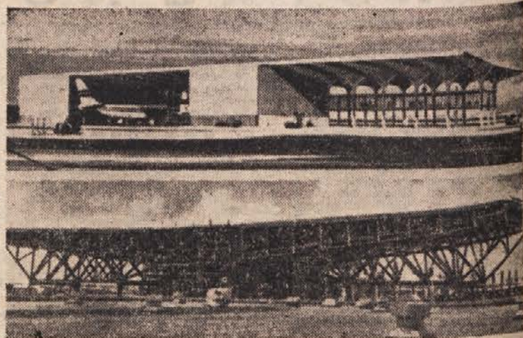
Svojevrsen hangar za šest velikih transportnih letal DC-8 gradijo na letališču pri Miamiu na Floridi. Krili segata na obe strani po 34 m daleč, poslopje je zgrajeno iz železobetona. Strokovnjaki pravijo, da bo streha vzdržala vihar s hitrostjo nad 300 km na uro, temelji pa so podobni tistim, kot jih uporabljajo na peščenih tleh.
