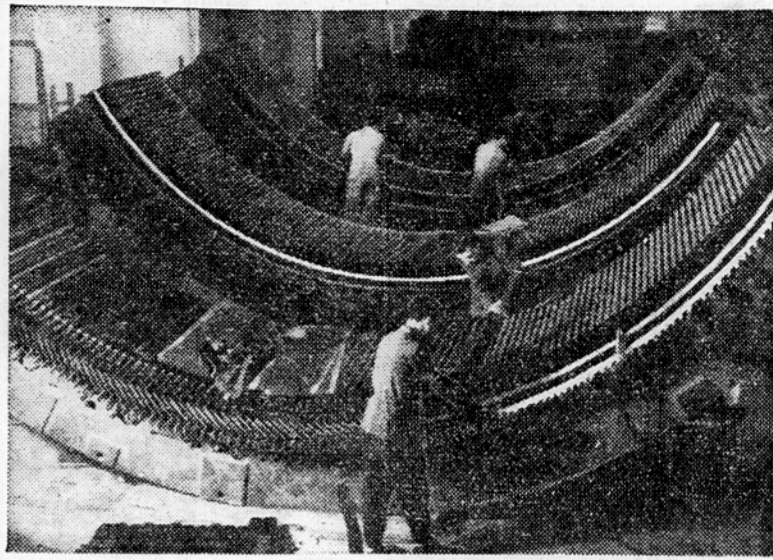
V tovarni »Rade Končar« bodo v kratkem dovršili tudi stator velikega generatorja za hidrocentralo v Vuzenici. Celotni generator tehta 215 ton, sam stator, razdeljen na tri dele, ki jih vidimo na sliki, pa 85 ton.
