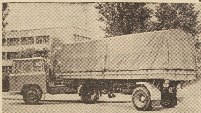
Novo vozilo TAM: vlačilec «TAM 6500 BVL», nosilnost 12 ton; zračno hlajen Diesel motor 125 KS. Izdelava kabine «Avtomontaža» Ljubljana, izdelava prikolice «Itas» Kočevje.
