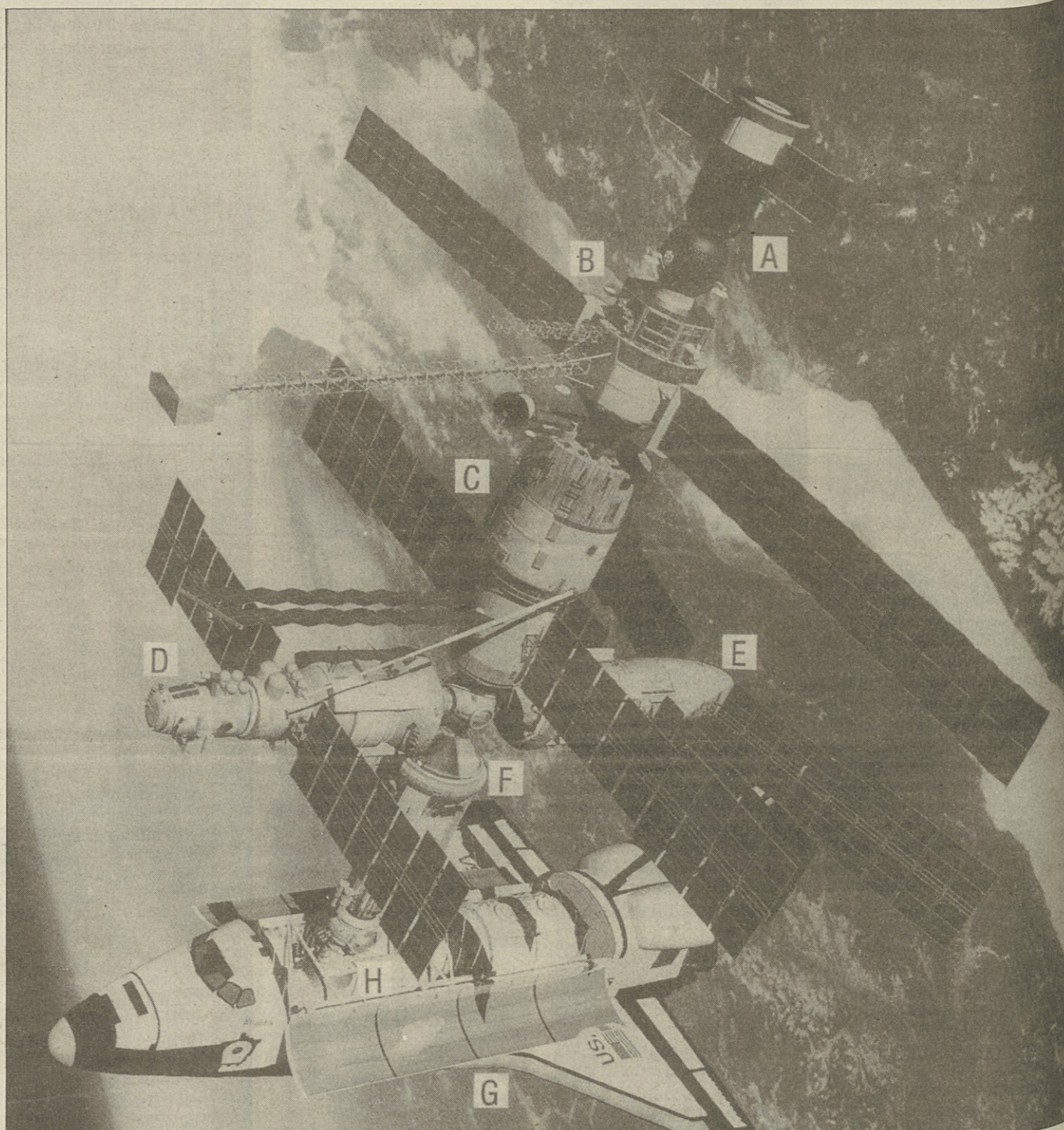
Slika zapletene planetarne postaje Mir in vesoljskega taksija Atlantis: a) Sojuz - trajektni modul, b) raziskovalna postaja Kvant, c) Komandni odesek, d) poskusni laboratorij Kvant-2, e) merilna postaja Spekter, f) Kristal z izmenjevalnikom energije, g) Atlantis, h) pristajalni segment za Space shuttle
